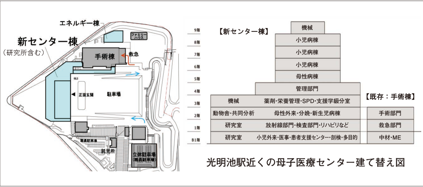
建物配置(左)と建物断面(どちらもイメージ)
